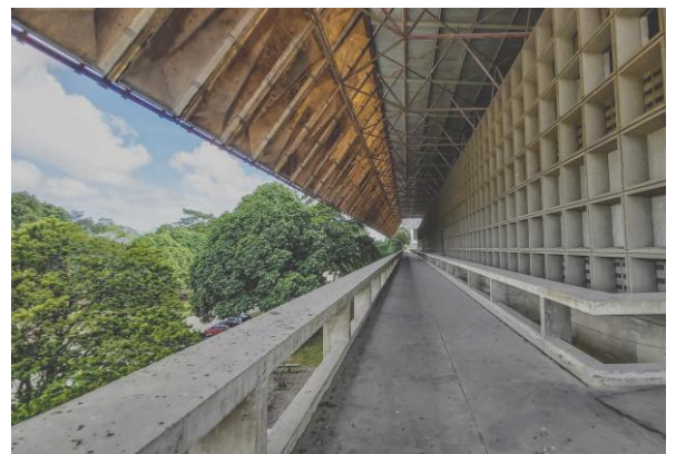
Detalhes construtivos da Fábrica Hering Nordeste em Paratibe, Paulista /PE.Fonte: Alcilia Afonso. 2022.
